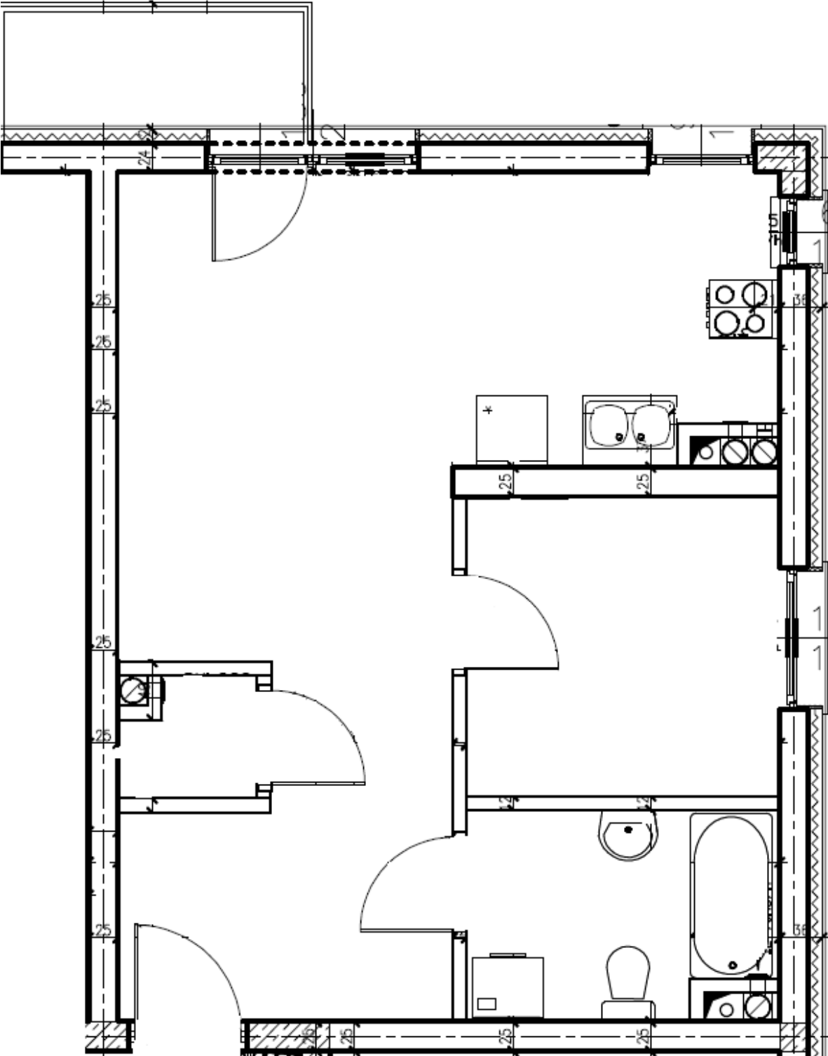
Rzut mieszkania ul. Wileńska 15
